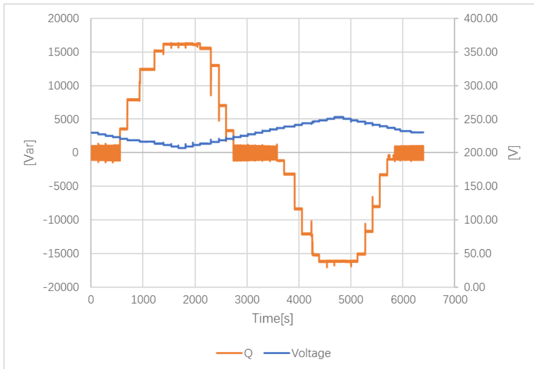
Q(U) Diagram
