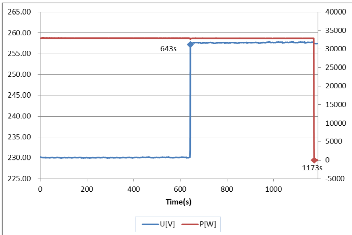
Un to 112% Un
